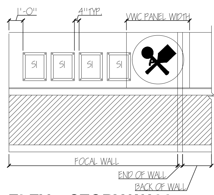
1 ELEV. - STORY WALL A-7 SCALE: 1/4" = 1'-0"
